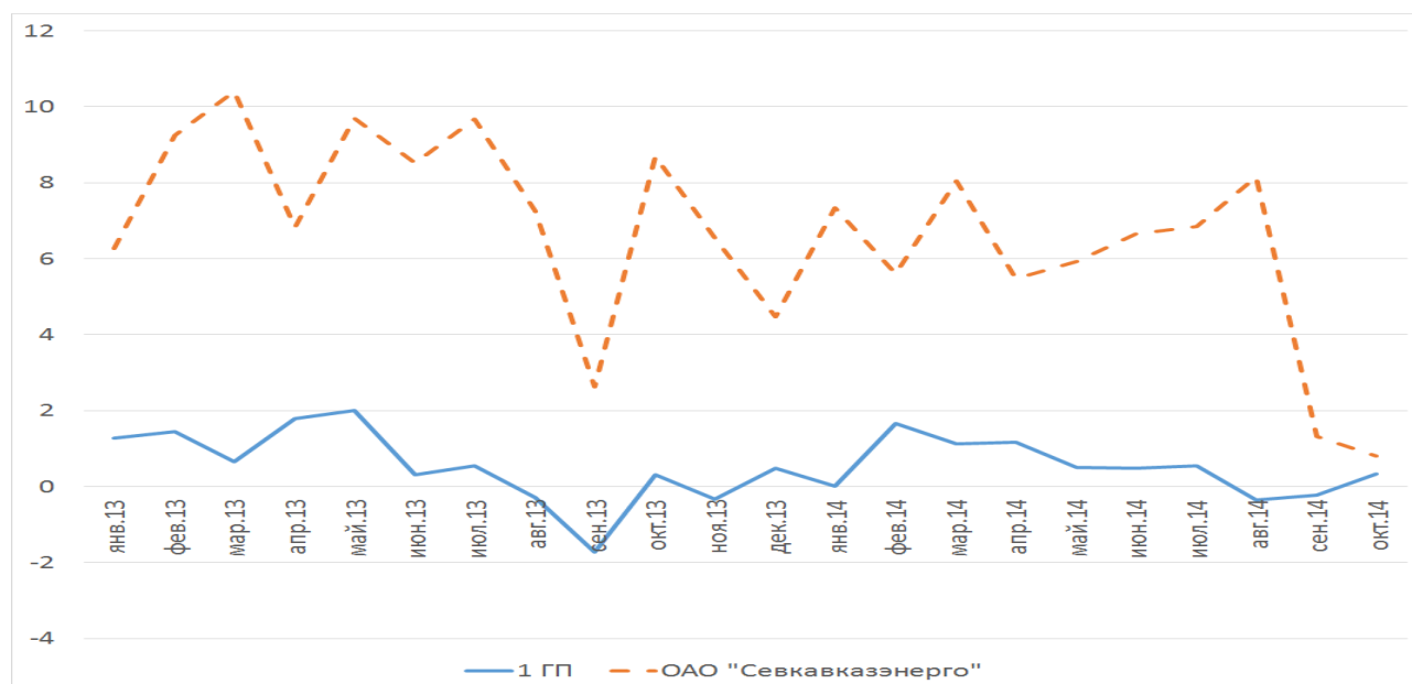
График 6 Статистика отклонений от планового потребления ОАО «Севкавказэнерго» (%)
