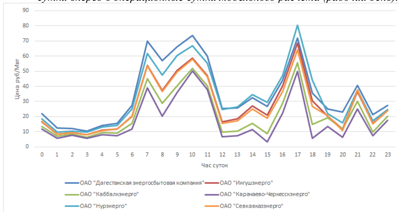
График 7. Почасовая статистика изменения равновесных цен рынка на сутки вперед в операционные сутки модельного расчета (рабочий день).
